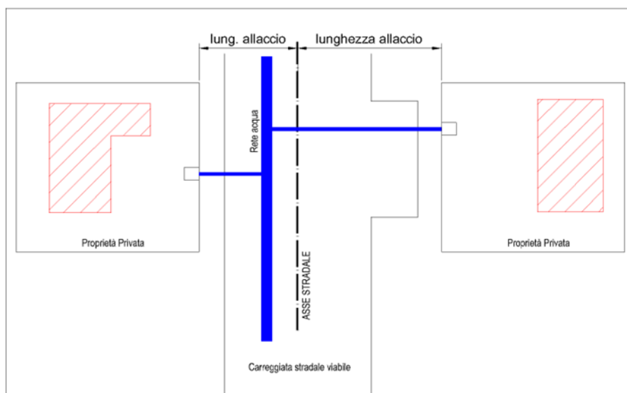
Figura 2 – misura della lunghezza di allacciamento
