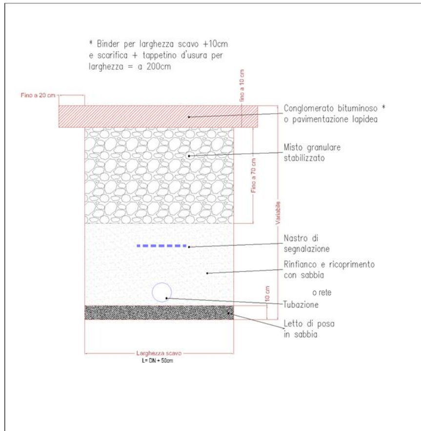
Figura 3 - Parametri standard allacciamento
