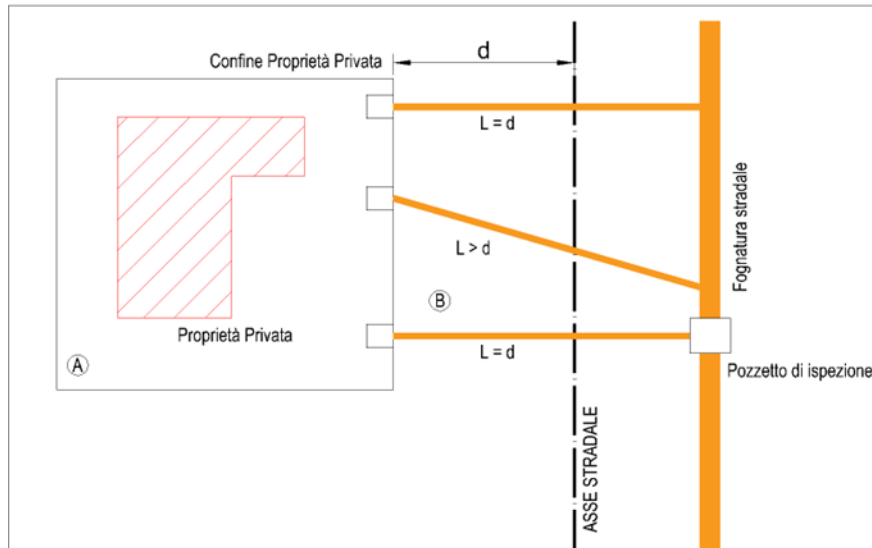
Figura 1 – misura della lunghezza di allacciamento
